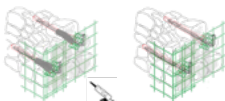
5 POSIZIONAMENTO DEL FAZZOLETTI, INSERIMENTO ED ANCORAGGIO CHIMICO DEI CONNETTORI
