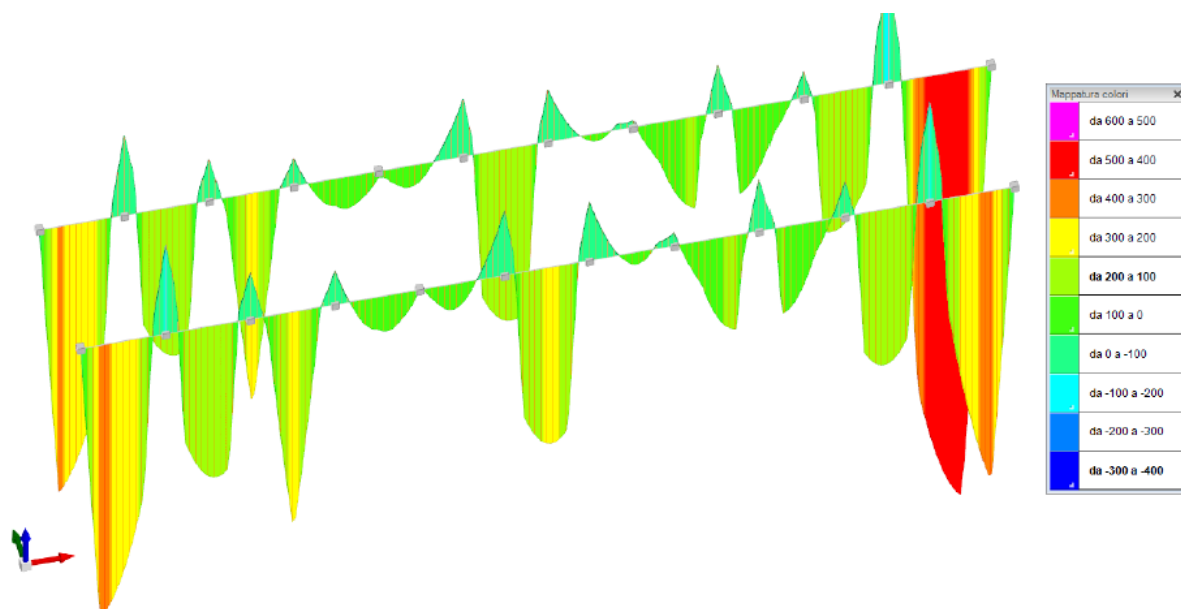
Figura 14: Involuppo momento M3 - Valori massimi
