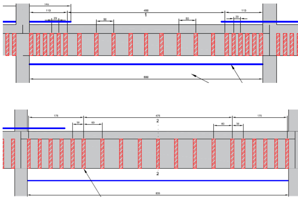
Figura 3 Campate travi tipologia C (sezione di riferimento n°2)
