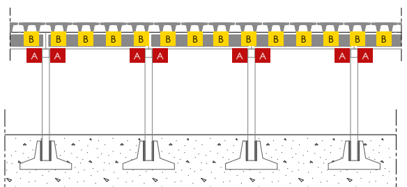
Struttura monopiano con copertura piana con elementi a forma alare
