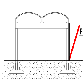
Ribaltamento del tamponamento
