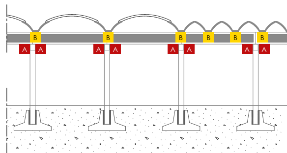
Struttura monopiano con copertura piana discontinua
