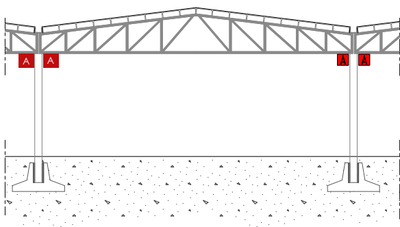
Struttura monopiano con travi di copertura reticolari
