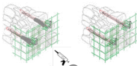
5 POSIZIONAMENTO DEL FAZZOLETTI, INSERIMENTO ED ANCORAGGIO CHIMICO DEI CONNETTORI
