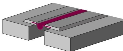
Schema di applicazione per elevati movimenti di lavoro
